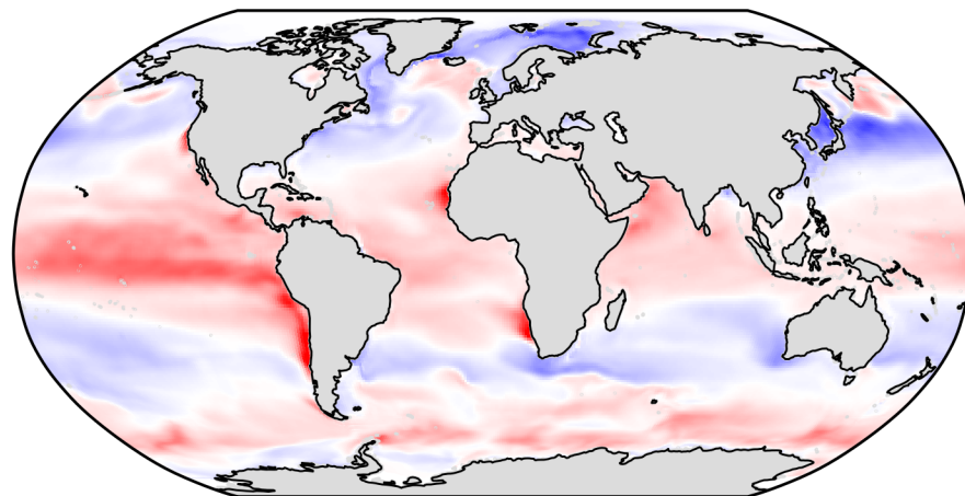
air-sea CO2 flux
