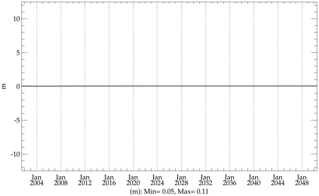
hic005 (20010101 - 20501231) Global Mean SSH
