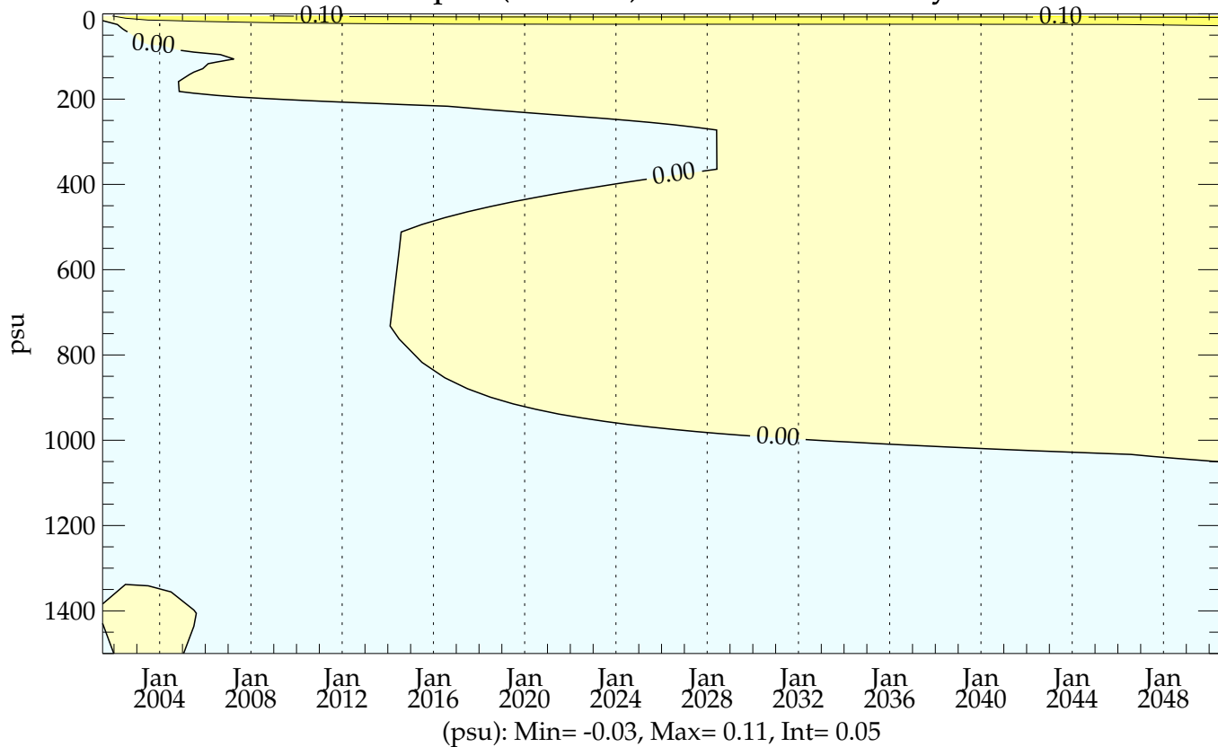
hic005 (20010101 - 20501231) - Levitus ZT-plot (0-1500m) Global Mean Salinity
