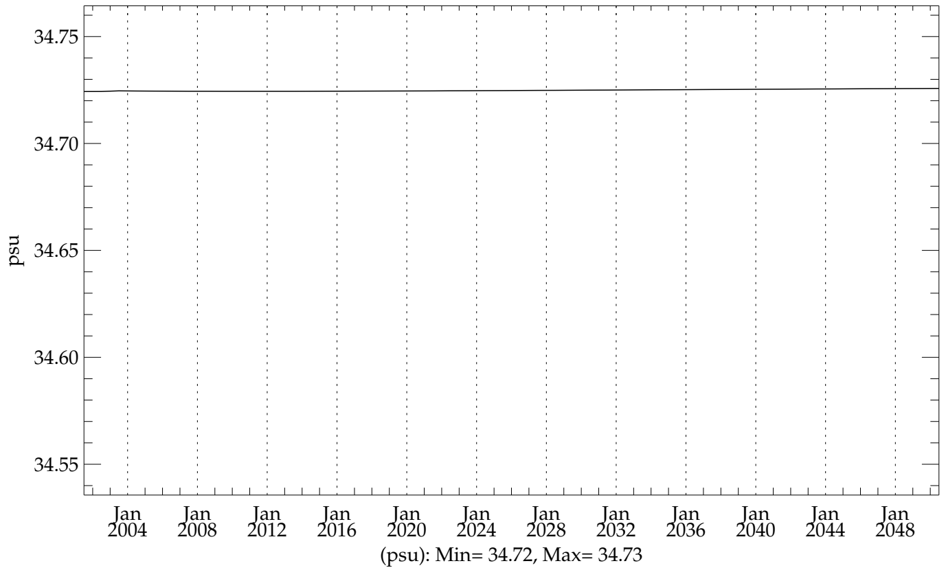
hic005 (20010101 - 20501231) Global Mean Salinity
