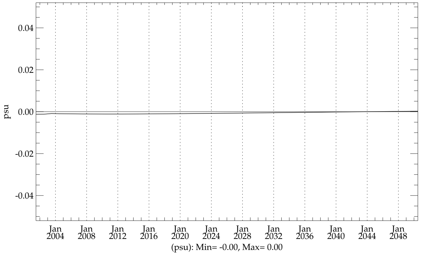
hic005 (20010101 - 20501231) - Levitus Global Mean Salinity
