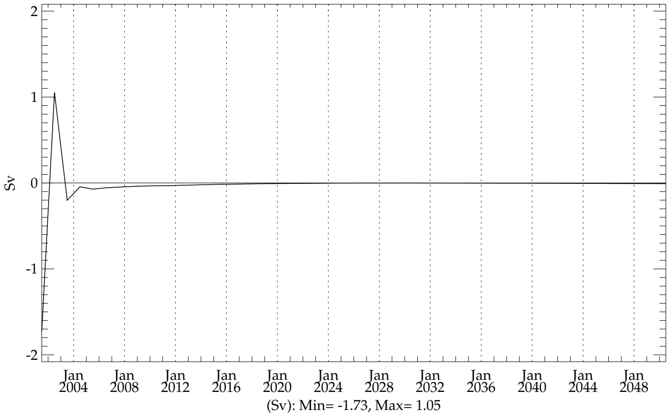
hic005 (20010101 - 20501231) Global Mean EMP
